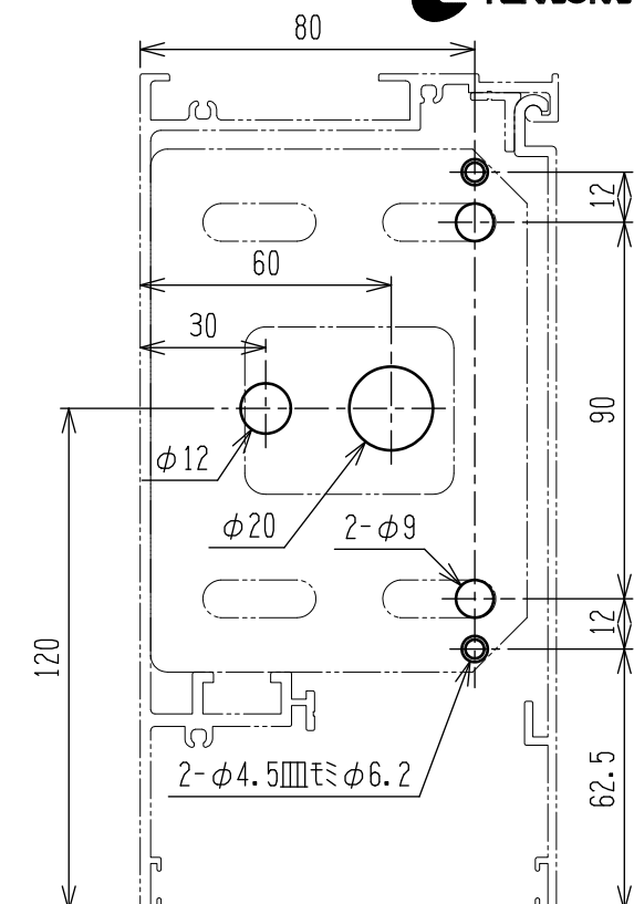
△ Fフロント フェイシングフロント (SG) 100見込 (上框隠蔽・細見付たて框 CF9)
