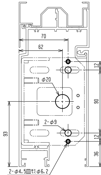
SYSTEMA 520e (複層) ランマ無
