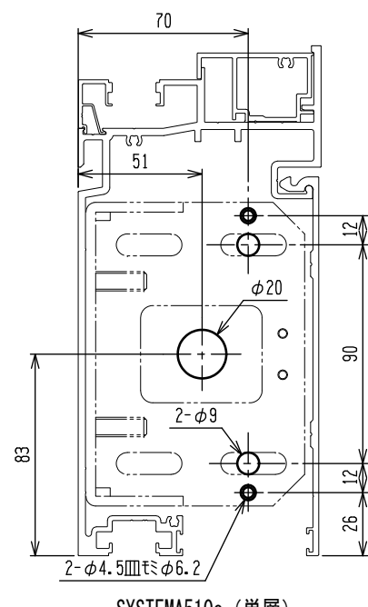
SYSTEMA510e (単層) ランマ有
