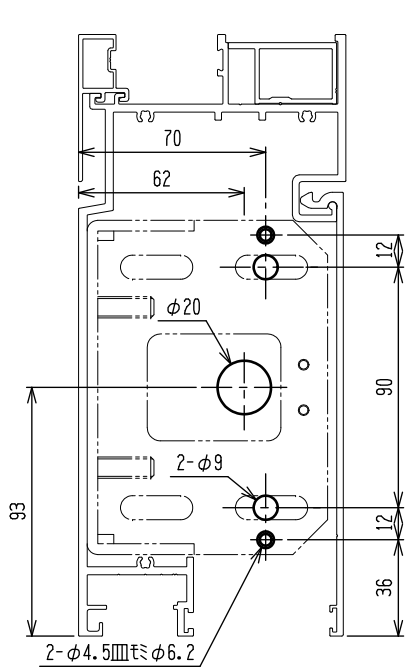
SYSTEMA 520e (複層) ランマ有
