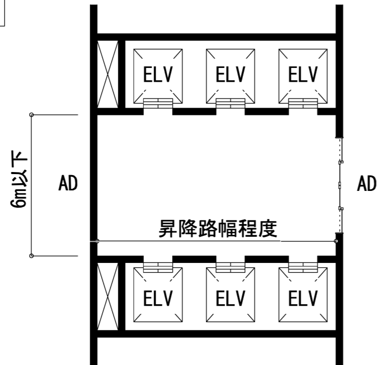
パターン図 3
