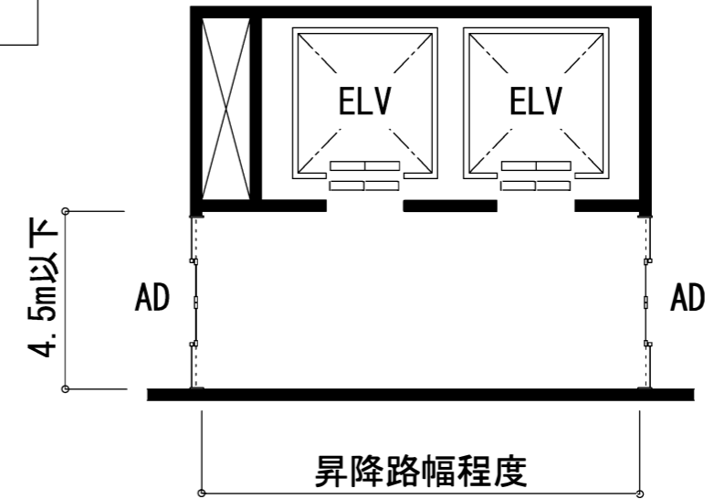
パターン図2
