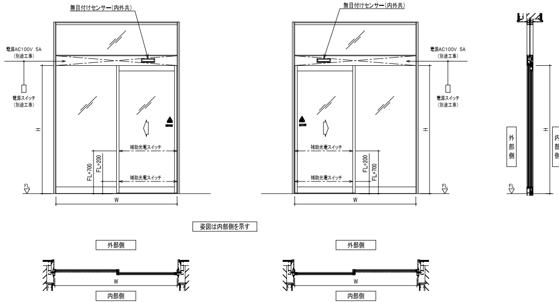
よこ断面詳細図
