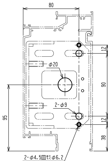
Fフロント フェイシングフロント (PG) 障子36mm・FIX部36mm硝子溝
