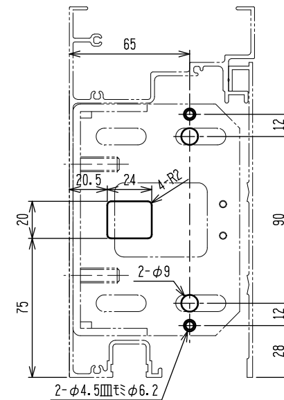
Fフロント フェイシングフロント (SG) 150見込
