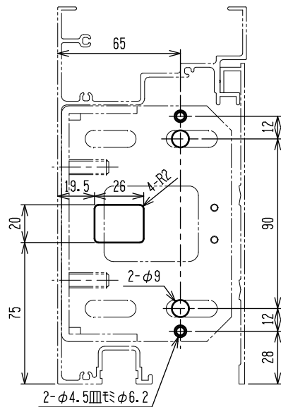
Fフロント フェイシングフロント (SG) 100見込 (ランマ無し)
