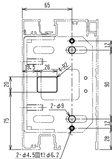
Fフロント フェイシングフロント (SG) 100見込 (ランマ有り)
